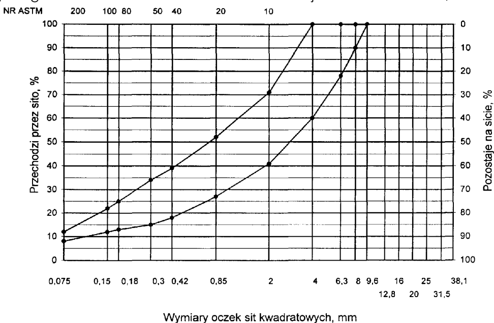
warstwy ścieralnej nawierzchni drogi o obciążeniu ruchem KR1 lub KR2 Rys. 3. Krzywe graniczne uziarnienia mieszanki mineralnej BA od 0 do 8mm, od 0 do 6,3 mm do warstwy ścieralnej nawierzchni drogi o obciążeniu ruchem nawierzchni drogi o obciążeniu ruchem KR1 lub KR2
